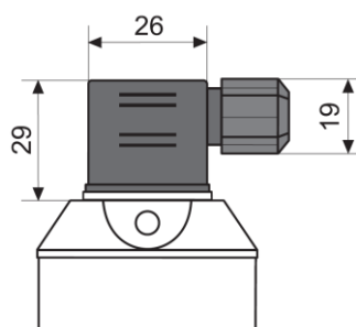
DIN 43650A
